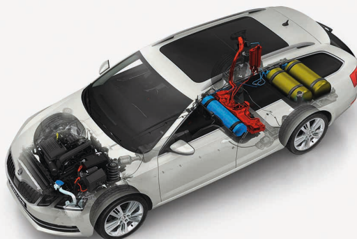
Moteur d'une Skoda Octavia G-TEC, avec les deux bonbonnes de gaz à l'arrière. © SKODA AUTO
